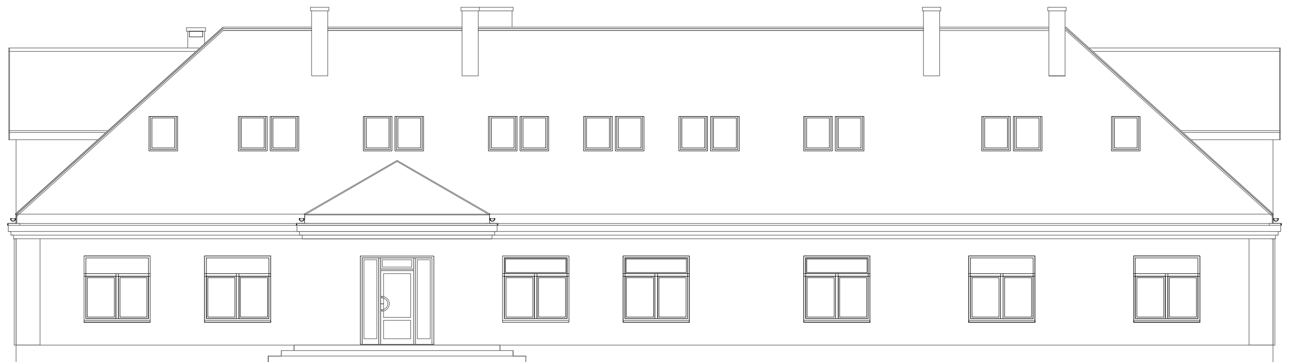
ELEWACJA FRONTOWA - PÓŁNOCNA
